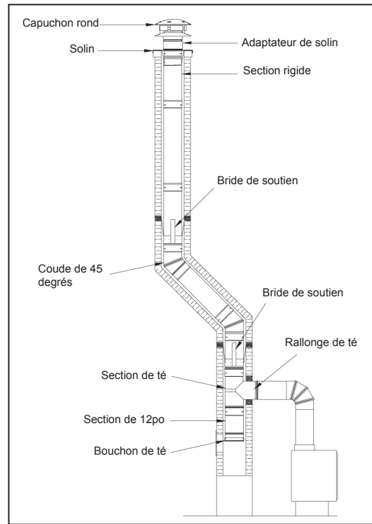
Installation typique du conduit rigide en acier inoxydable en décalage
