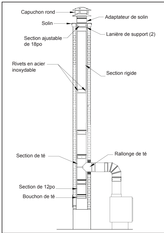
Installation typique du conduit rigide en acier inoxydable
