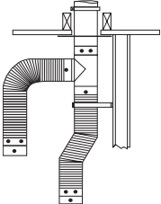
DÉCALAGE TRAVERSANT LE PLAFOND
