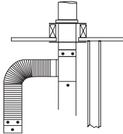
DÉCALAGE 90° AVEC TÉ
